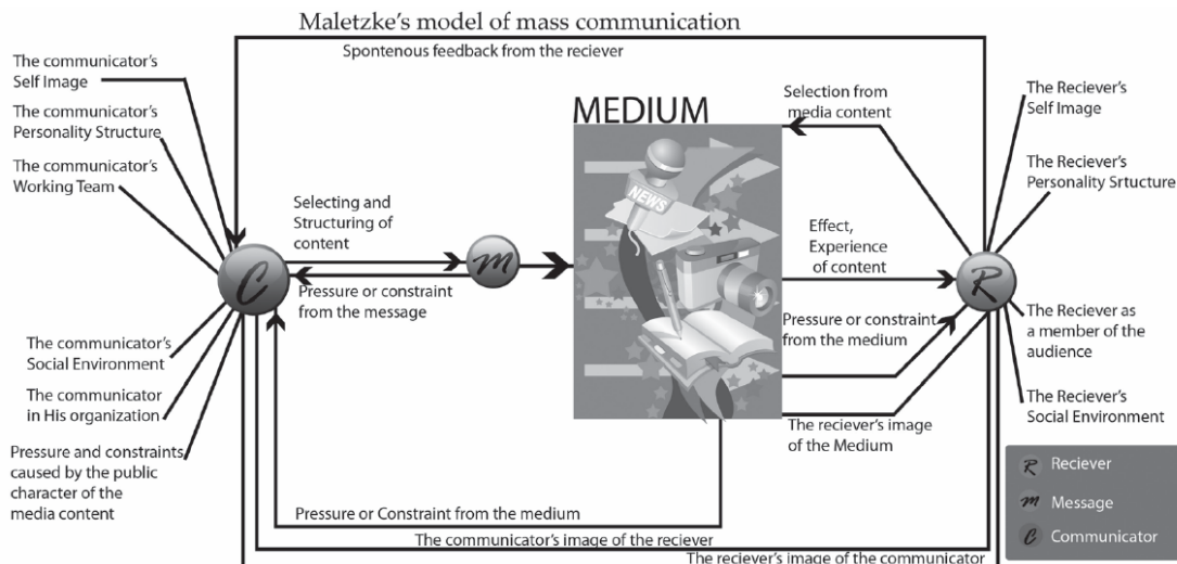
Figura 3 – Modelul Maletzke
