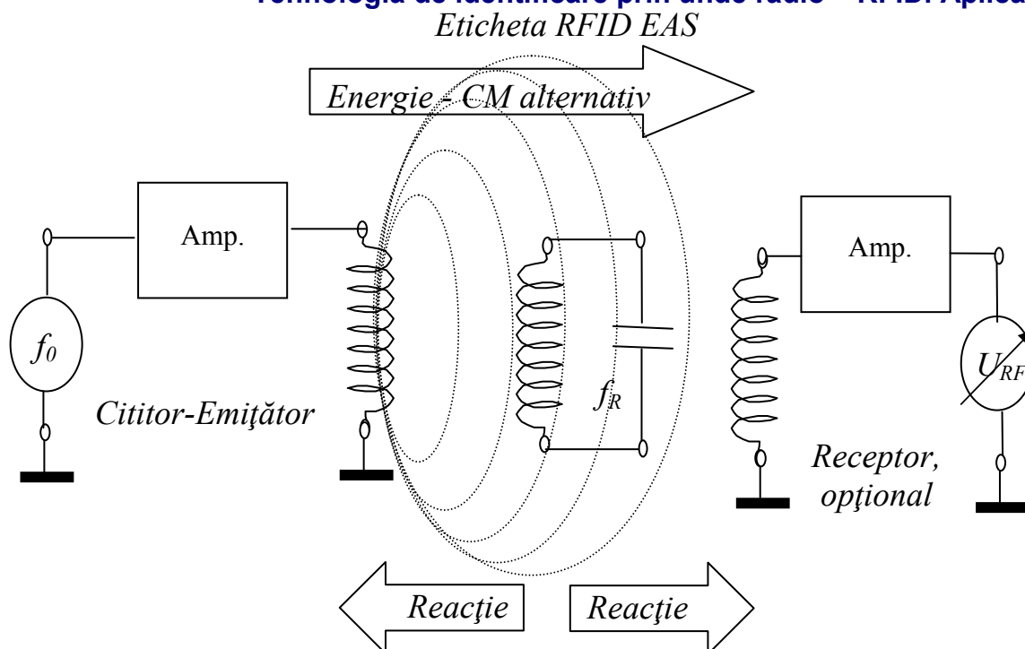
Figura 3.2 Principiul detecției prezenței etichetei EAS prin cuplaj RF
