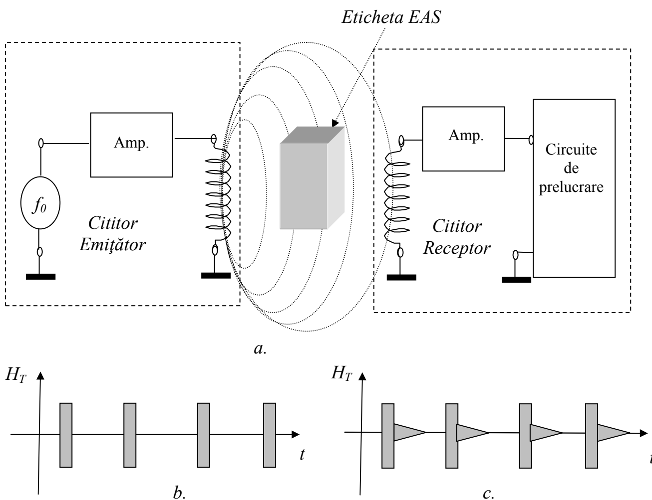
Figura 3.7 Sistem de securitate magnetostriktivă (a); variația câmpului magnetic fără (b) și cu (c) eticheta în aria de acoperire
