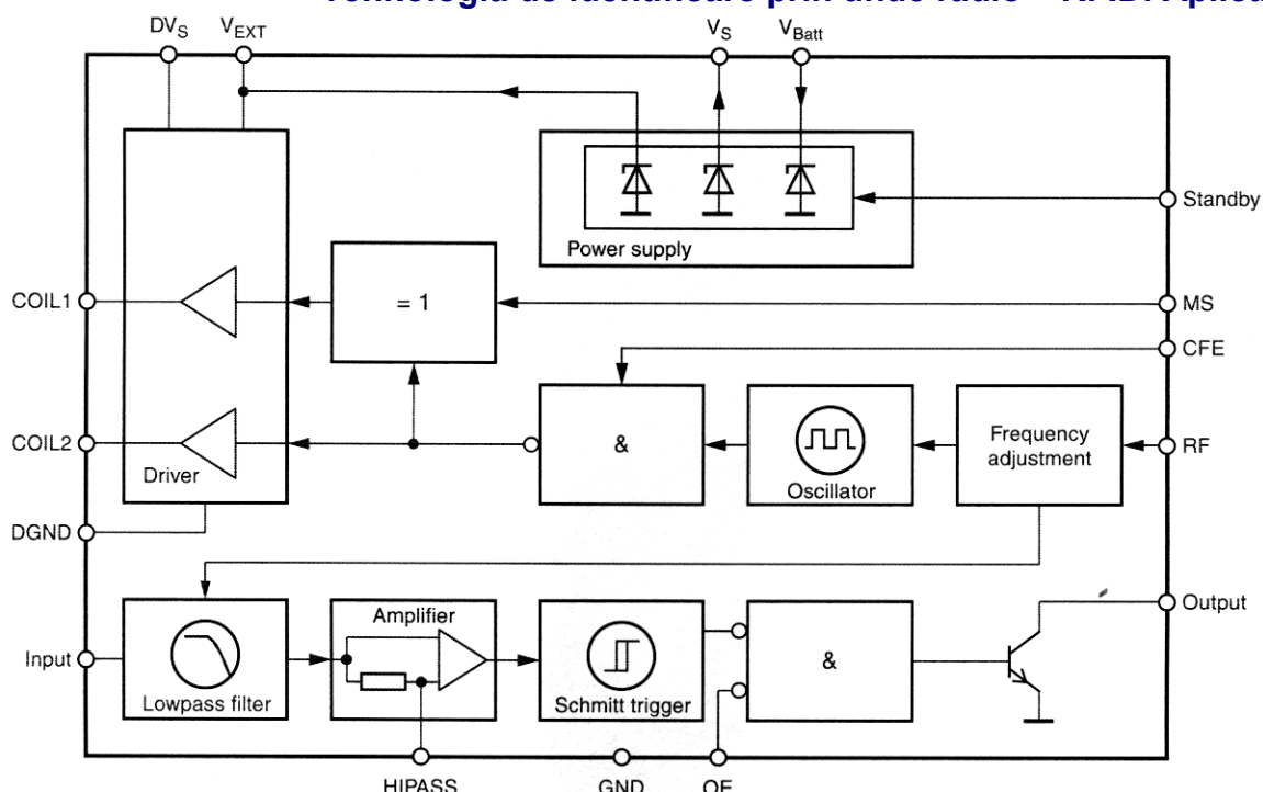
Figura 6.4 Schema bloc a CI U2270B
