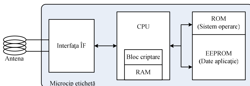
Figura 6.7 Schema bloc a unei etichete RFID cu microprocesor
