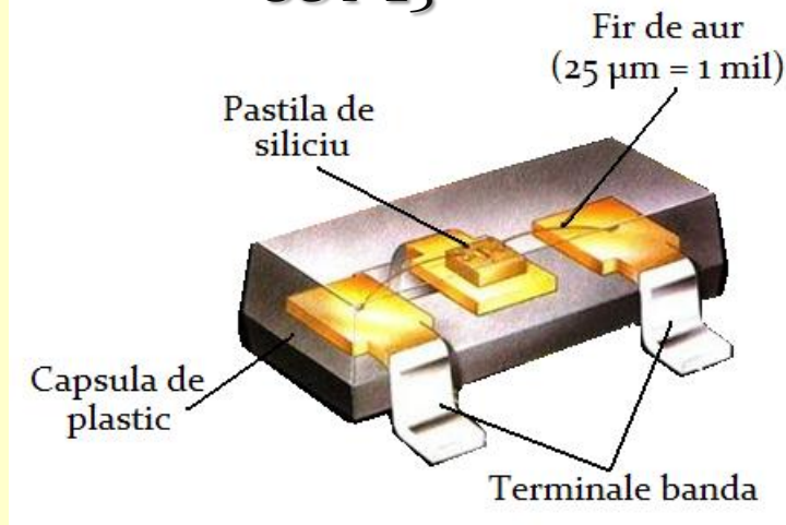
SOT-23
